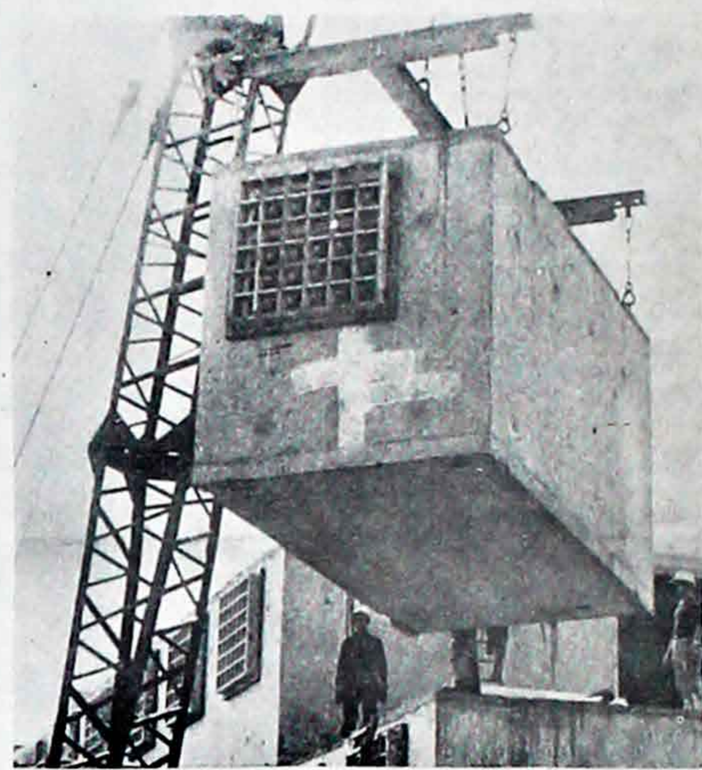
CARCEL DE CELDAS PREFABRICADAS - La cárcel más moderna de Europa se compondrá de celdas prefabricadas, de una superficie básica de 4,15 x 2,15 metros, las que se construyen al pie de la obra de hormigón que seca rápidamente. Cada celda pesa 12 toneladas y está equipada con cama plegable, mesa, silla WC, lavamanos, ventilación, calefacción central, luz y radio, así como una gran ventana enrejada.
