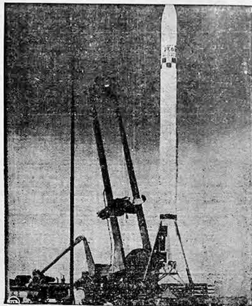
EL PROYECTIL GUIADO LLAMADO EL "CABO" APARECE cuando era preparado para ser disparado en los terrenos de prueba de White Sands en el Estado de Nueva México. Es una arma de superficie que puede destruir blancos fáciles a distancias mayores de 32 kilómetros que es el alcance del cañón atómico de 280 milímetros. — (U.P.)
