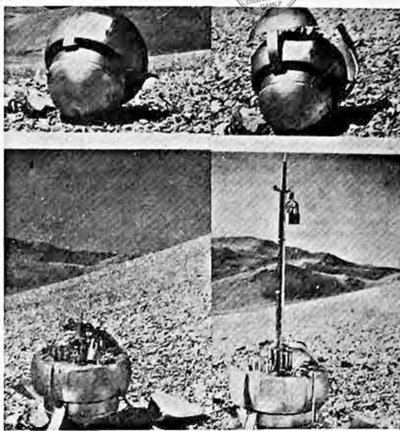
Es uno de varios aparatos que se perfecciona en los Estados Unidos para el Programa "Voyager" (viajero) de vehículos especiales sin tripulantes que explorarán a Marte en el decenio del año 1970.
