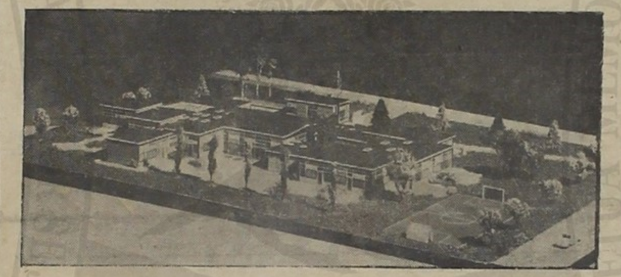
SISTEMA BRITANICO. — Modelo de una escuela que se erigió en Biella, Italia, por el método británico CLASP de construcción prefabricada. Este sistema se ha facilitado a Italia a raíz del éxito obtenido por la escuela primaria de un solo piso, exhibida en Gran Bretaña, en la duodécima trienal, el año pasado, construida con el mismo método.
